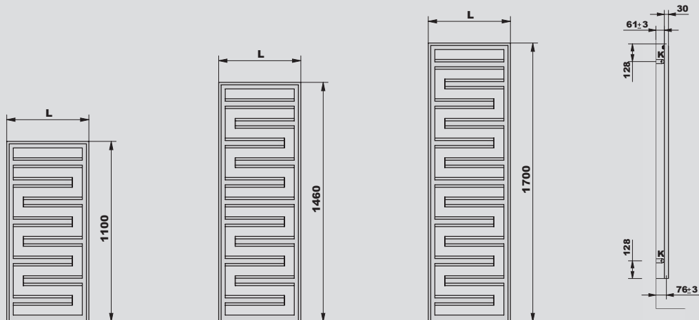
Schémas modèles eau chaude
